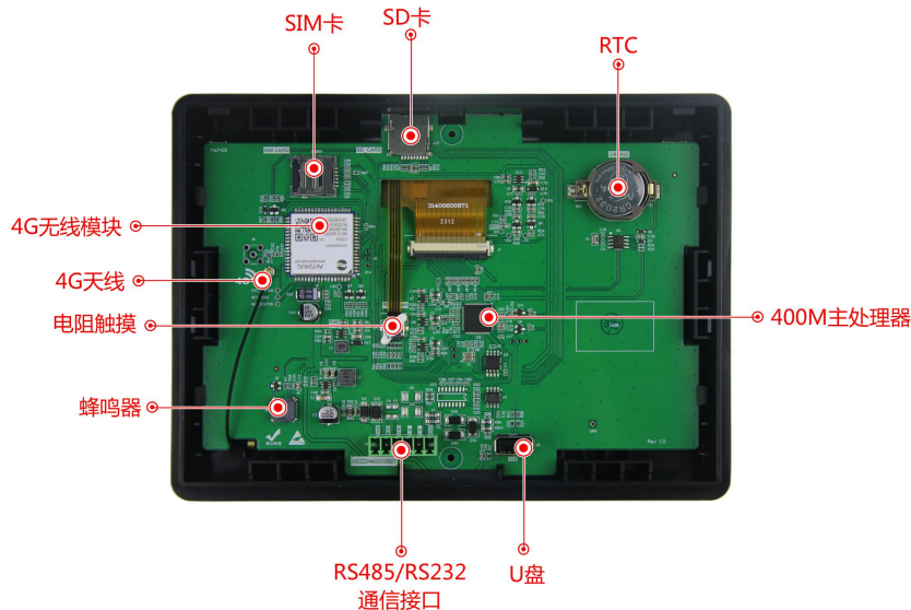
图 1-2 硬件配置图
