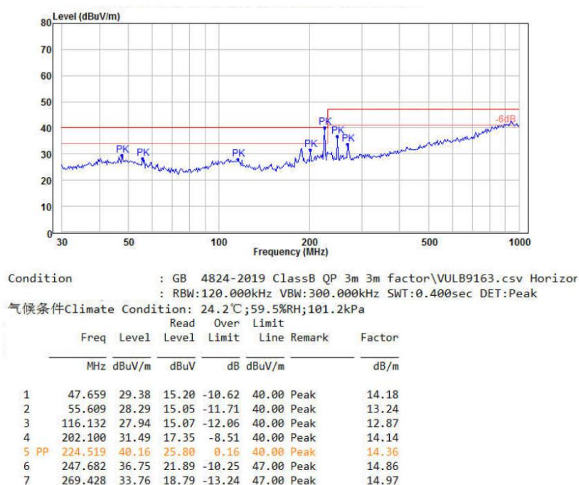
图 7-6 辐射测试水平方向
