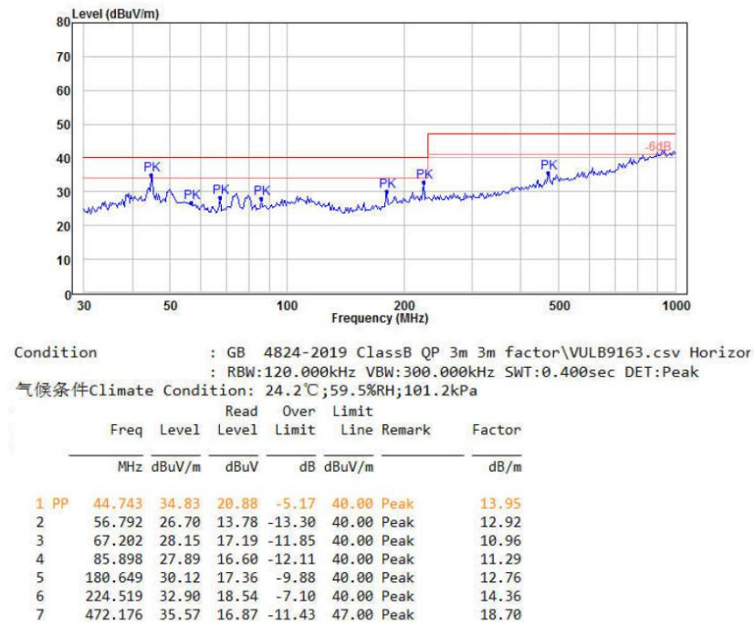
图 7-7 辐射测试垂直方向
