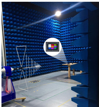
图 7-5 辐射测试图
